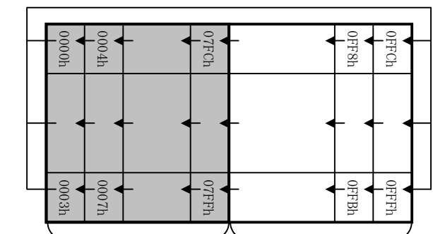
Display area 512dots Hidden area 512dots
