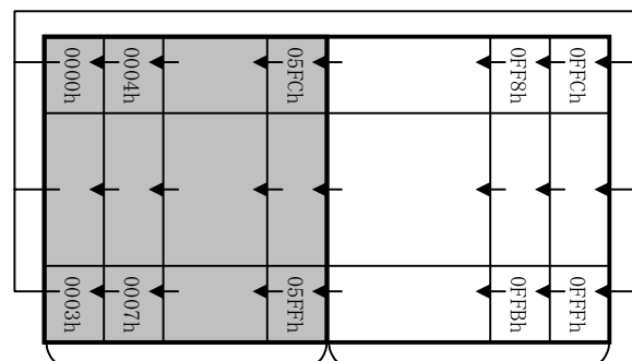
Display area 384dots Hidden area 640dots
