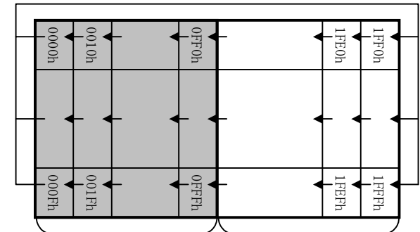
Display area 256dots Hidden area 256dots
